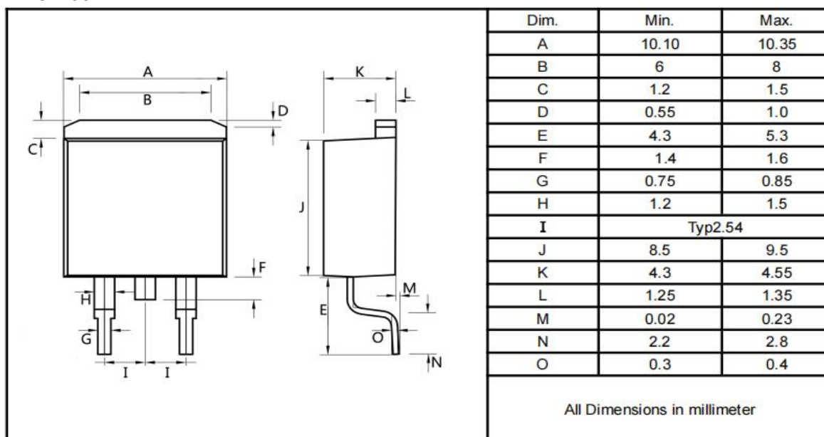
TO-263
